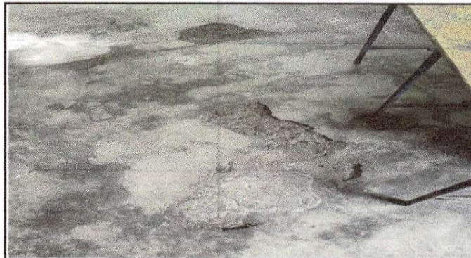
Foto 2: Sustrucción de piso de torta de concreto por piso cerámico ( 3 aulas y corredor)
