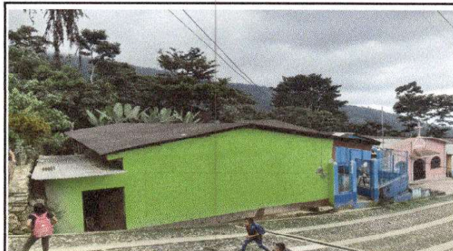
Foto 4: Sustrucción de lámina, por lámina troquelada aluzinc calibre 26. en establecimiento
